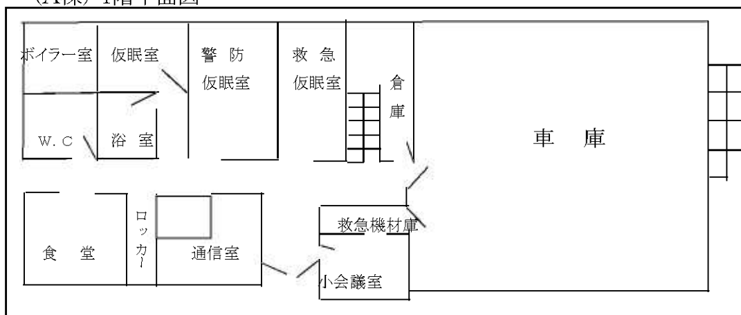
(A棟) 1階平面図
